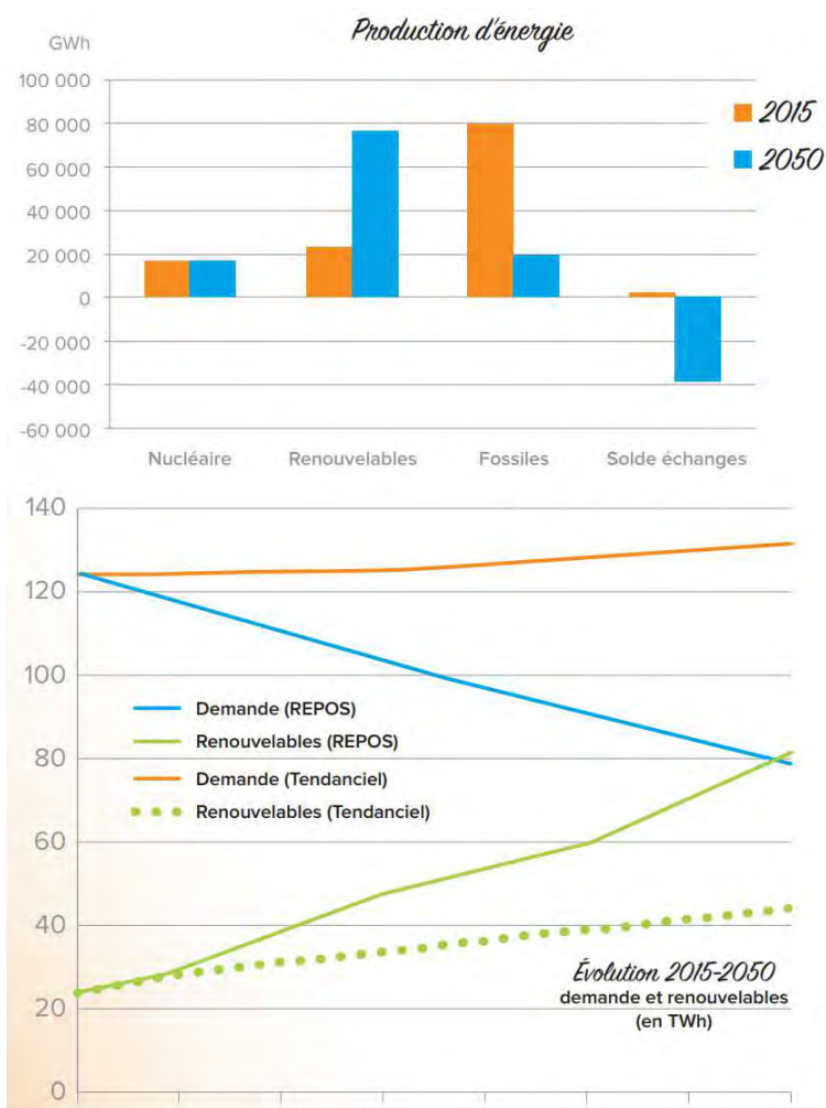
Figure 3 Evolution 2015-2050, demande et production d'énergie
